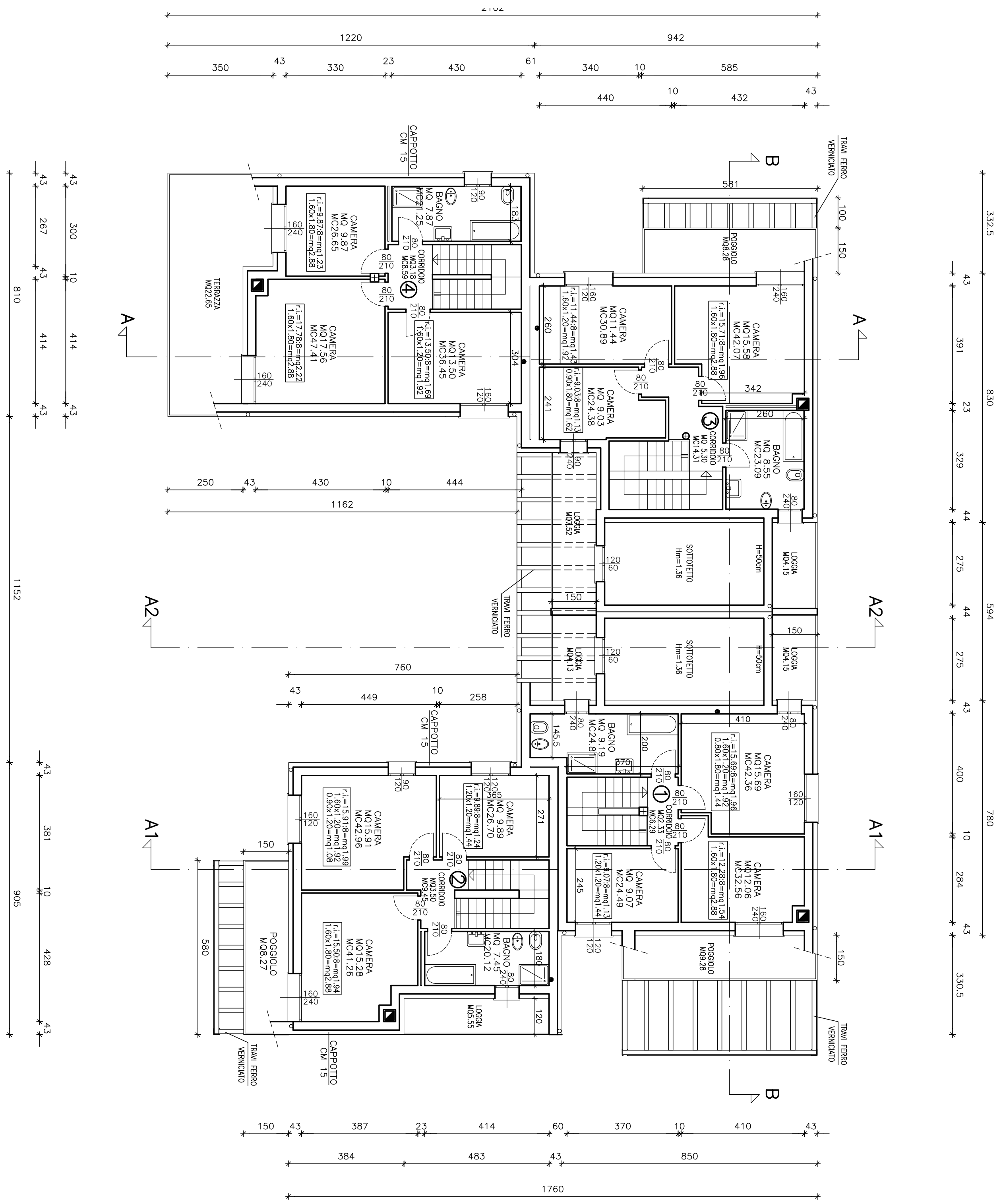
PIANTA PIANO PRIMO SCALA 1:100
